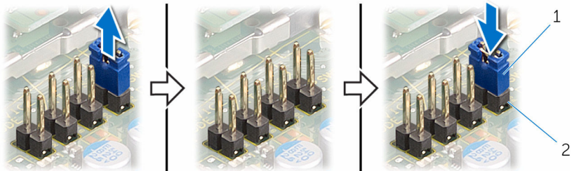
1 konektor prepojky
